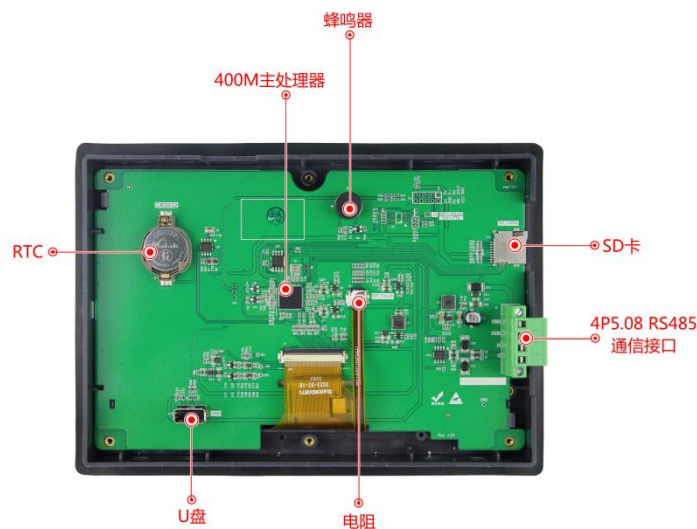
图 1-2 硬件配置图
